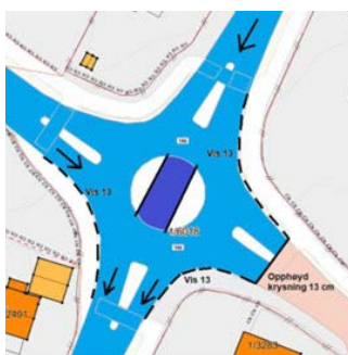
Figur 5.12: Flomvei gjennom rundkjøringens sentraløy med opphøyde krysningspunkter (Figur: [5.5]).
