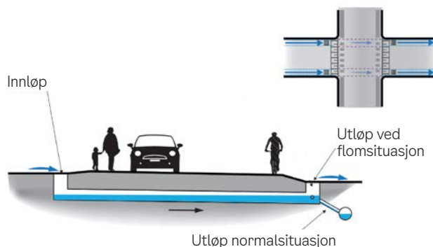
Figur 5.18: Flomveistunnel ved kryssende vei (Figur: Rambøll)
